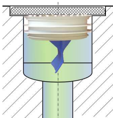
Przekrój instalacji zaworu w wpuście podłogowym
