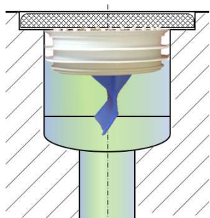
Przekrój instalacji zaworu w wpuszcie podłogowym
